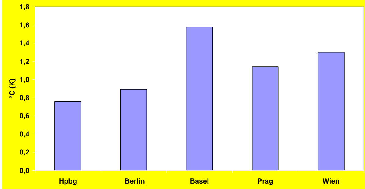
Abb.2 Temperaturanstieg an 5 Klimastationen Mitteleuropas 1851 - 2000
